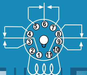
3PDT
